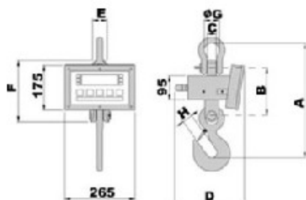
Wymiary wag MCW o nośności 150... 3000 kg oraz MCWT 6000 kg
