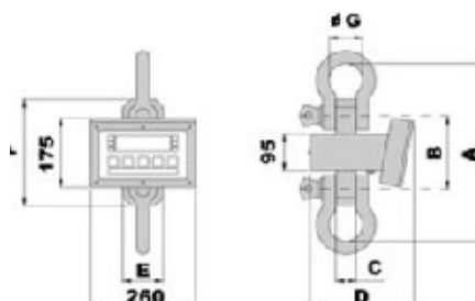
Wymiary wag MCWT o nośności 12... 25 t
