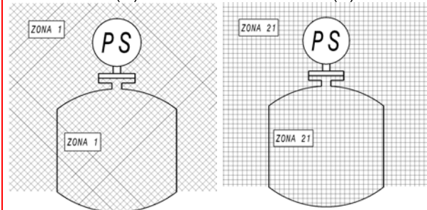
Fig. 6 - Installation of Group II Cat. 2 GD instruments Gas (G) Dust (D)
